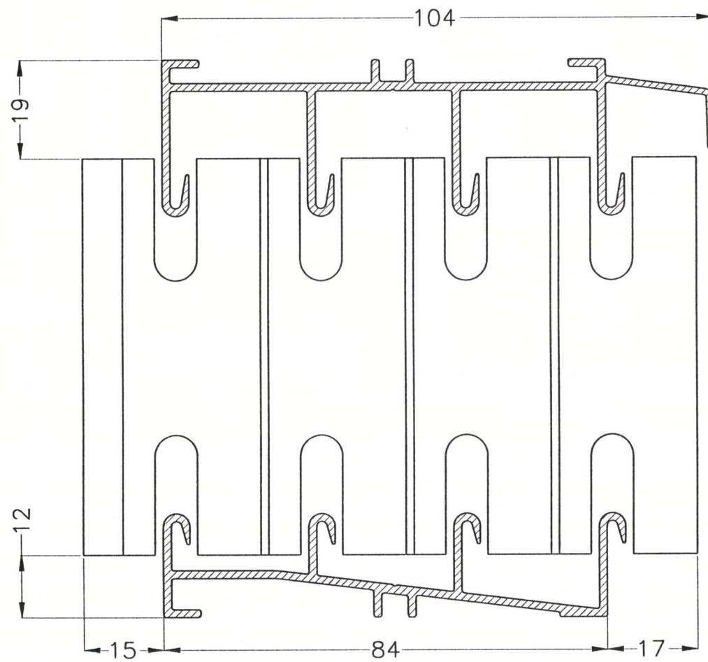
Måttuppgifter på 3&4 spårsskenor
